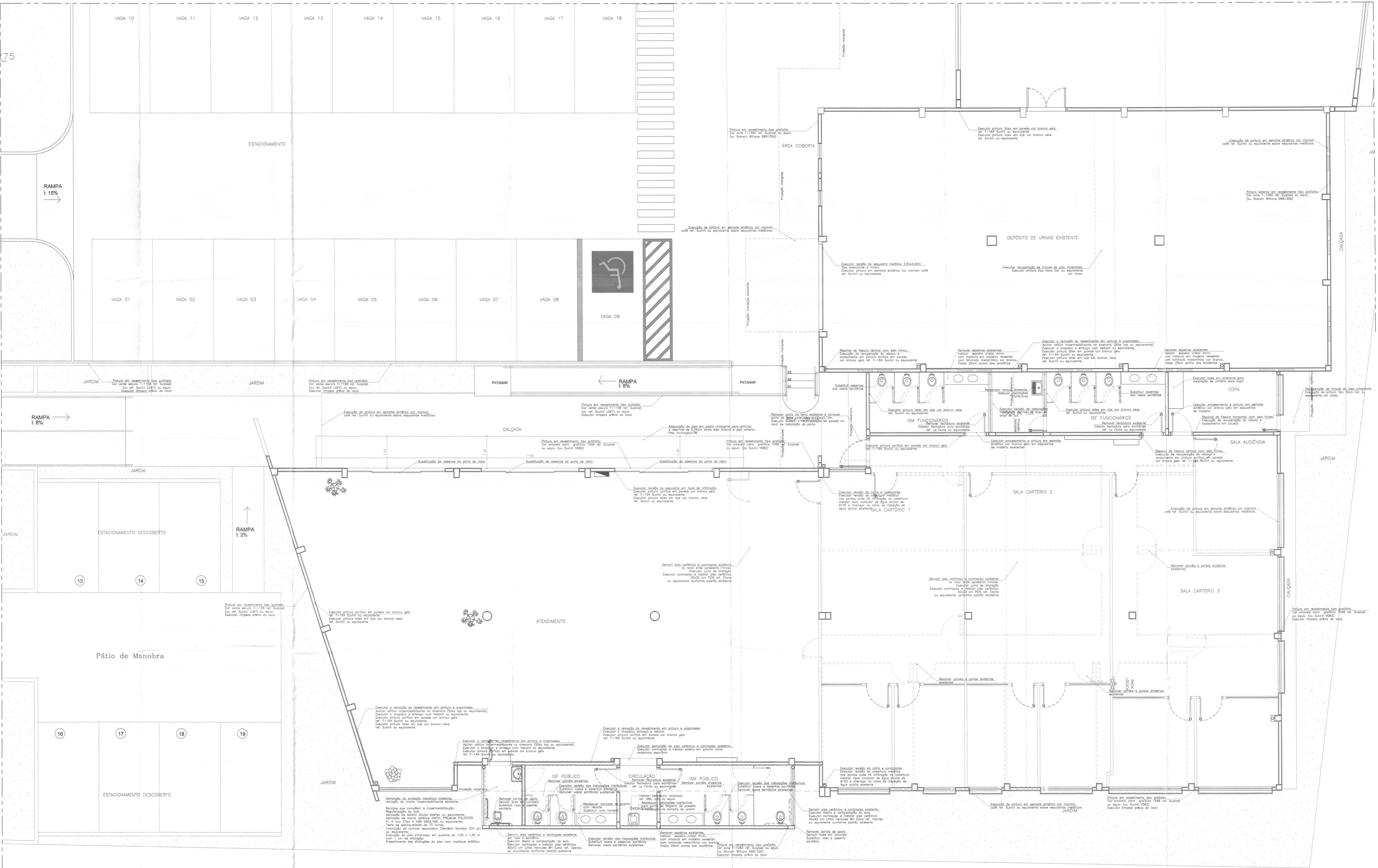
PLANTA ESC. 1:50
