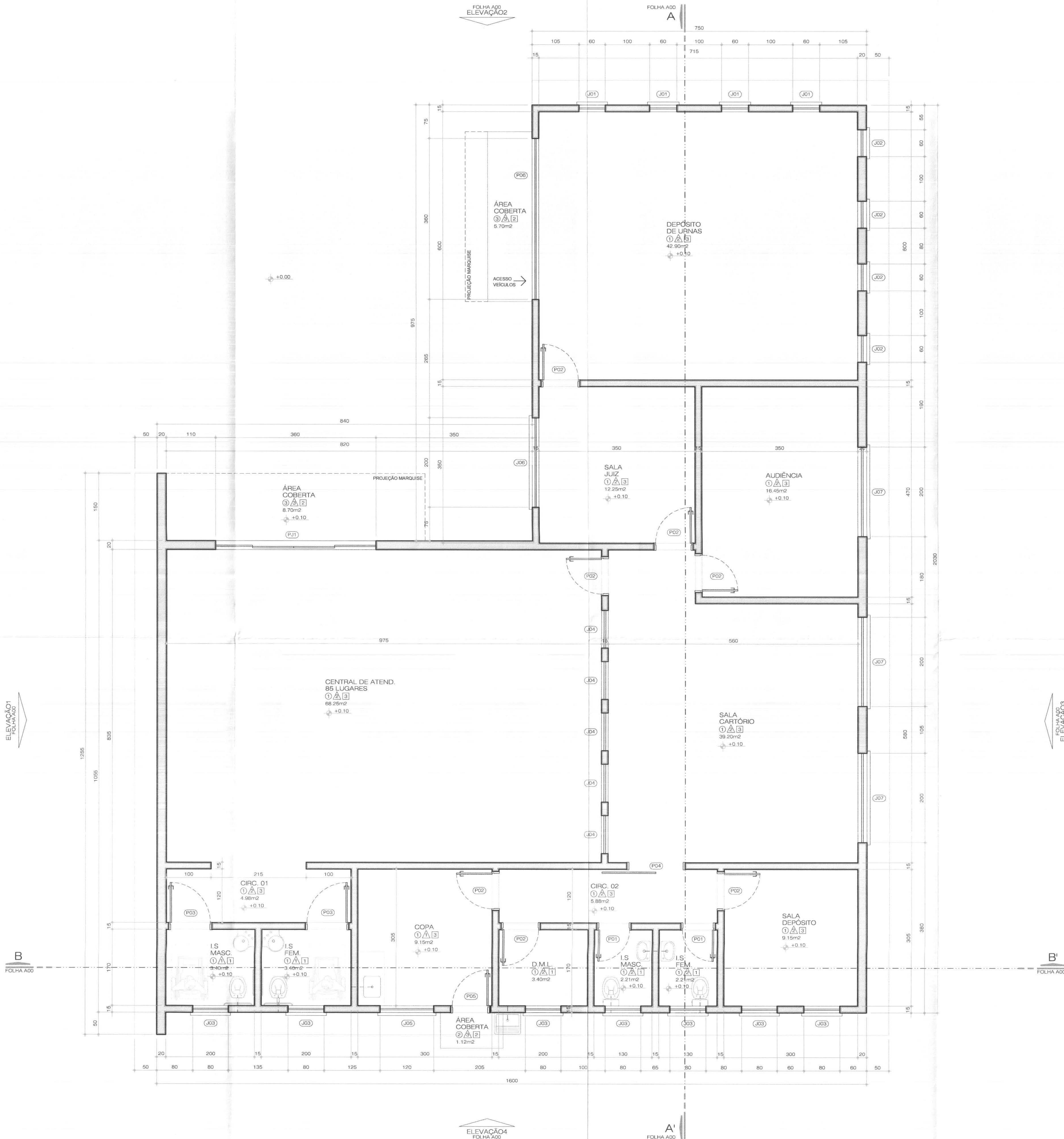
10 PLANTA PAVIMENTO TÉRREO ESCALA 1:50 A-240 86x47
