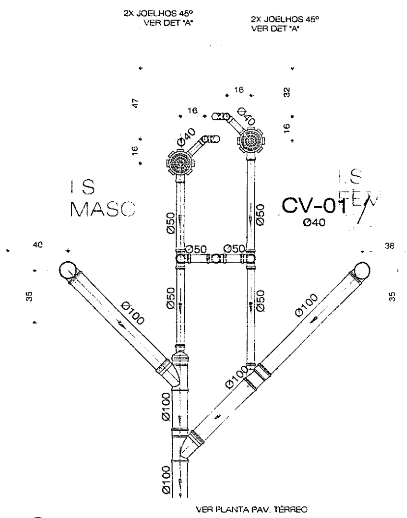
05 D 03 ESCALA 1:25
