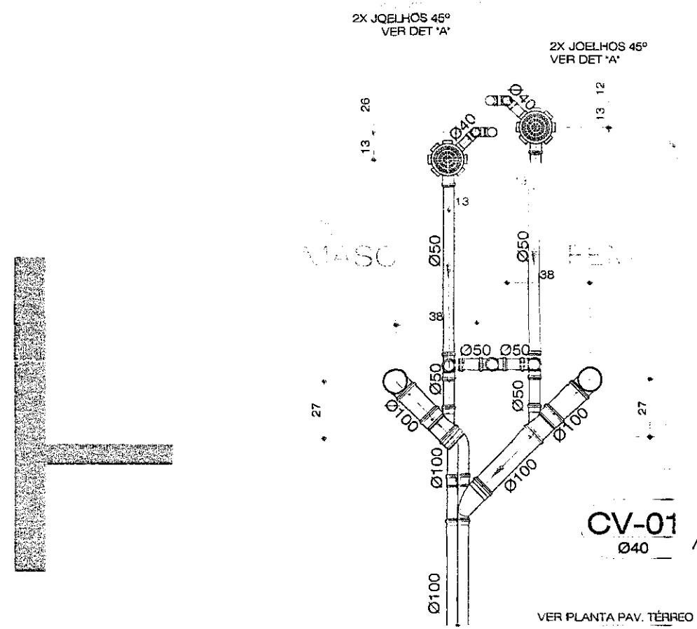
02 D 01 ESCALA 1:25
