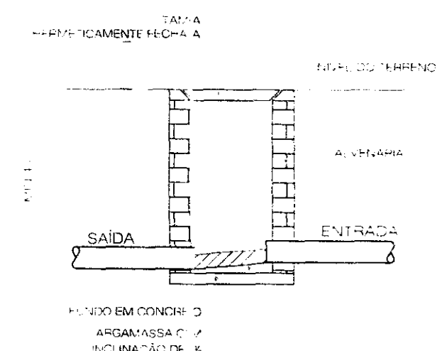
CORTE AA'
