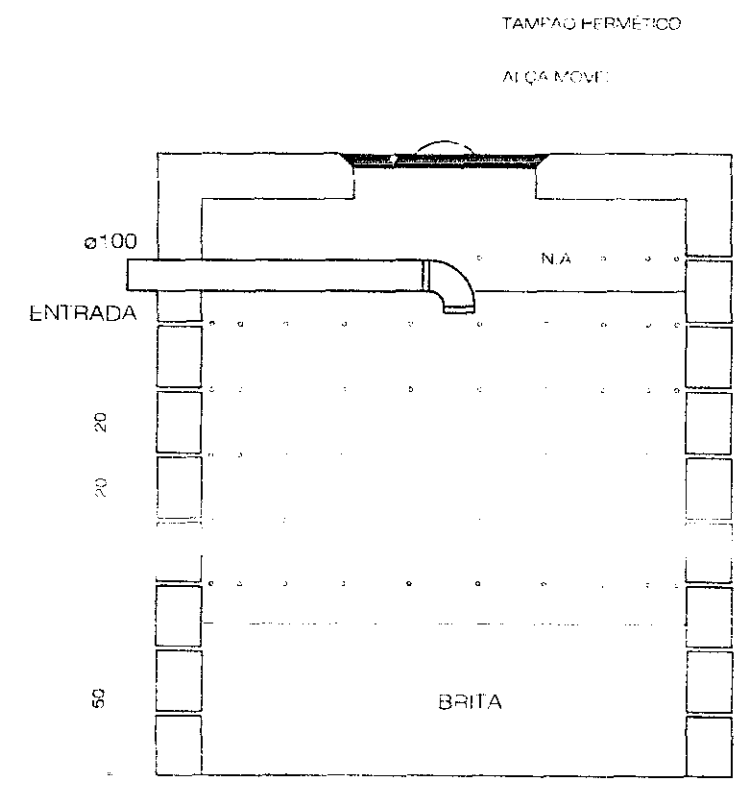
CORTE
