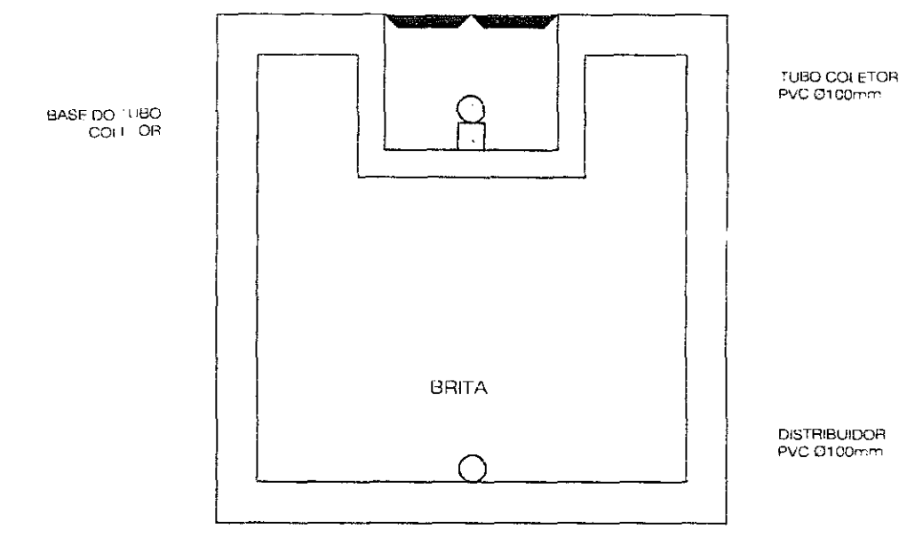
CORTE C
