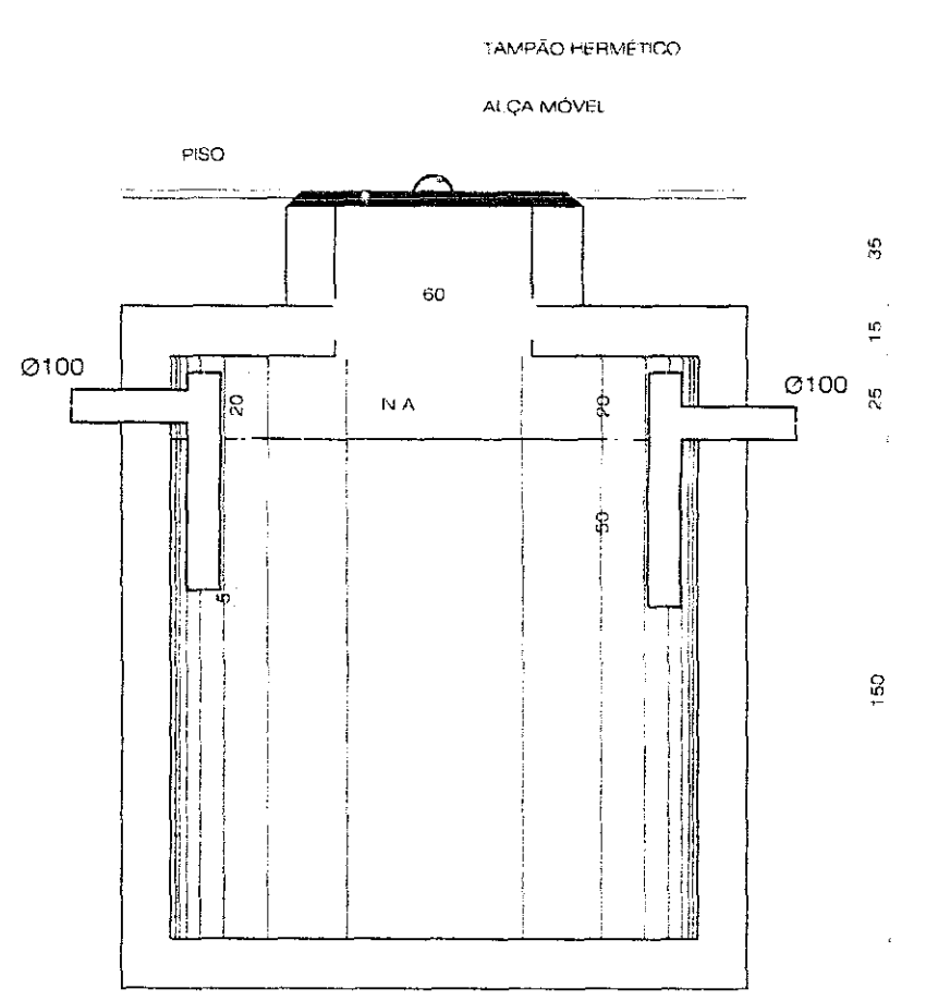
CORTE
