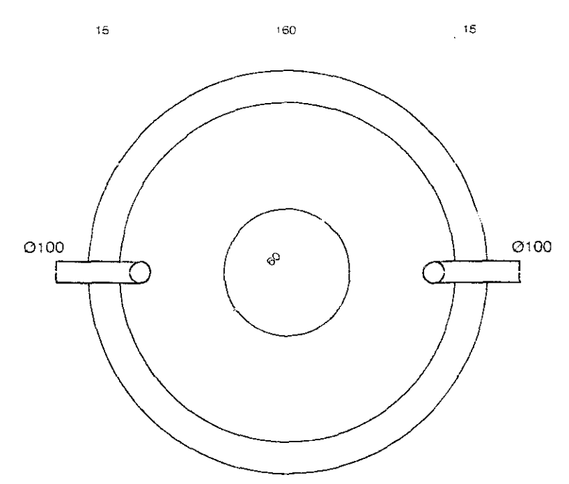
PLANTA BAIXA
