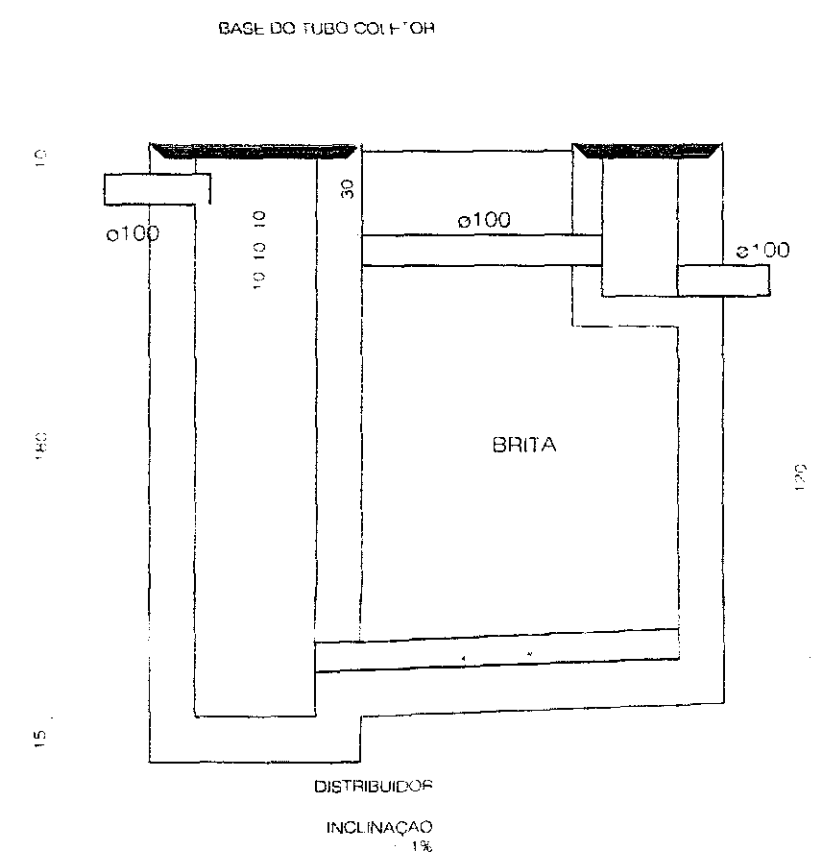
CORTE A
