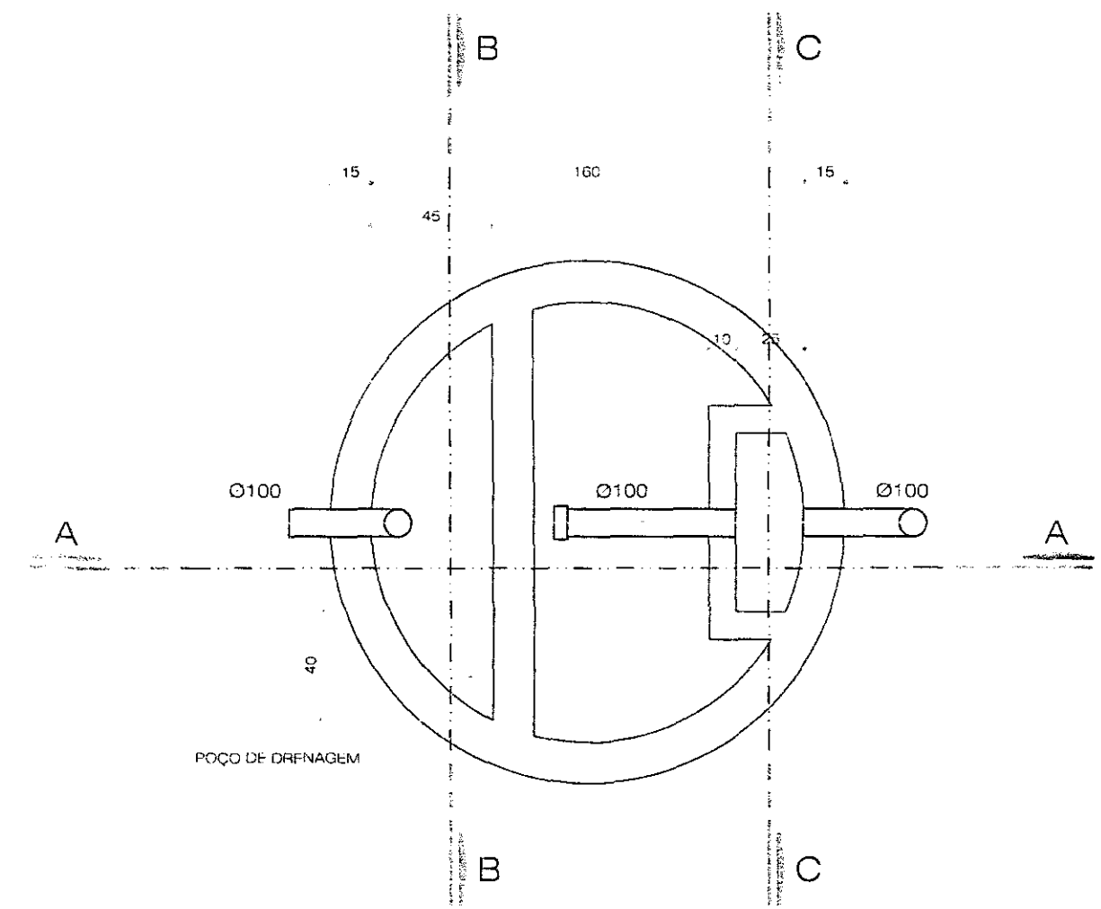
PLANTA BAIXA
