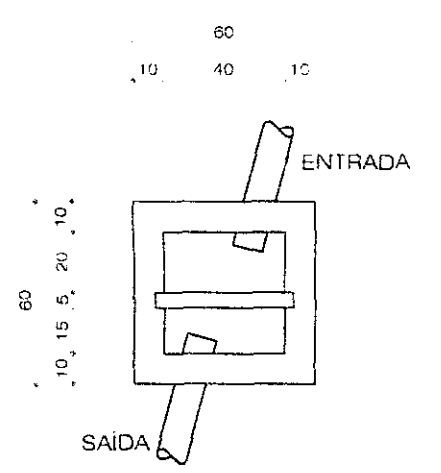
PLANTA BAIXA
