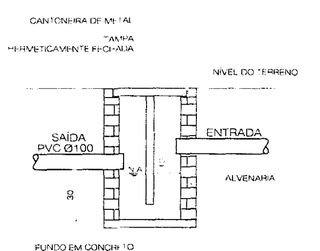
CORTE
