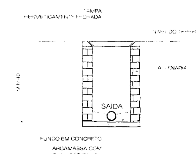
CORTE BB'
