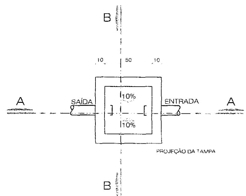
PLANTA BAIXA
